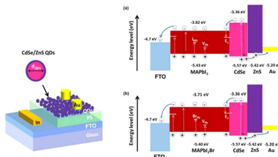
<CdSe/ZnS 양자점을 갖는 페로브스카이트 소자구조와 에너지밴드, 운반자 수송과정 모식도 >
