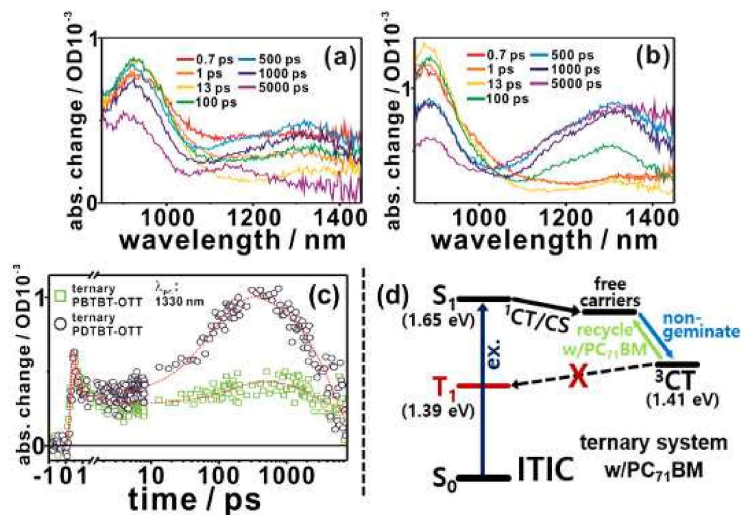
(a) PBTBT-OTT/PC71BM/ITIC 혼합 필름의 TAS. (b) PDTBT-OTT/PC71BM/ITIC 혼합 필름의 TAS. (c) 3차 혼합 필름의 TA kinetic profiles. 샘플은 1.6 μJ/cm 2 의 620nm에서 펌핑되고 1330nm로 조사되었다. (d) 3차 혼합 시스템에서 3CT 상태를 통과하는 전하-재활용 경로의 개략도.
